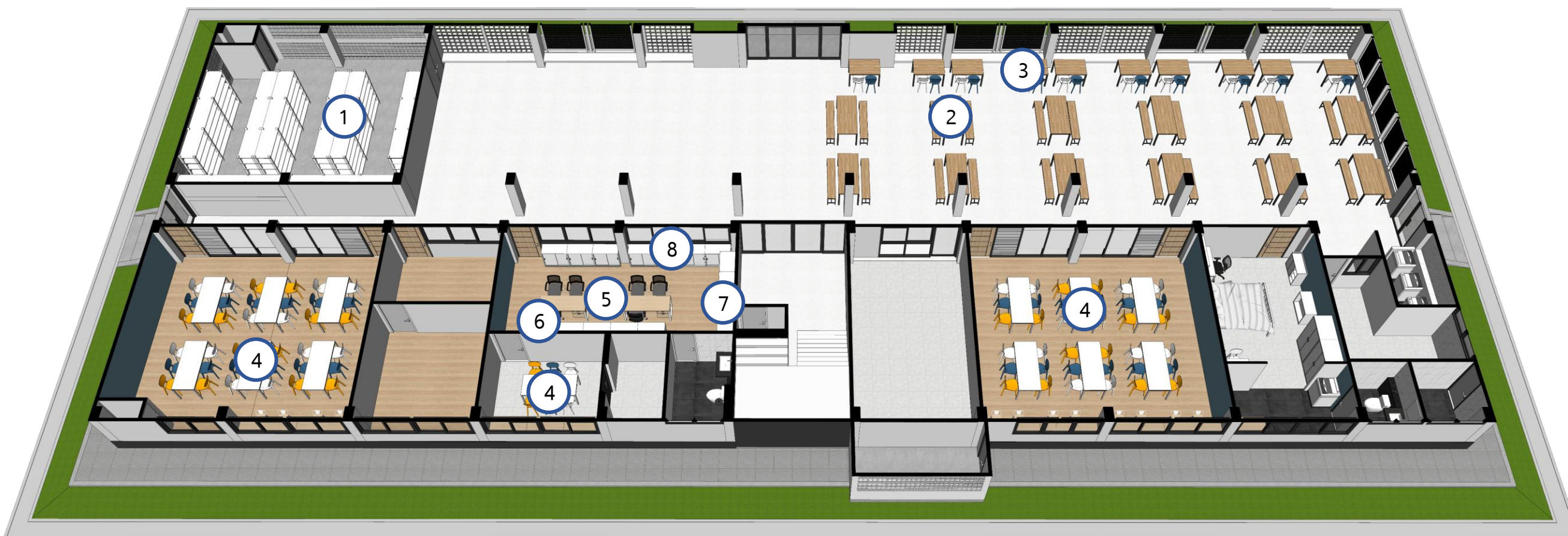
ผังพื้น ชั้นที่ 1 ( ISOMETRIC )
